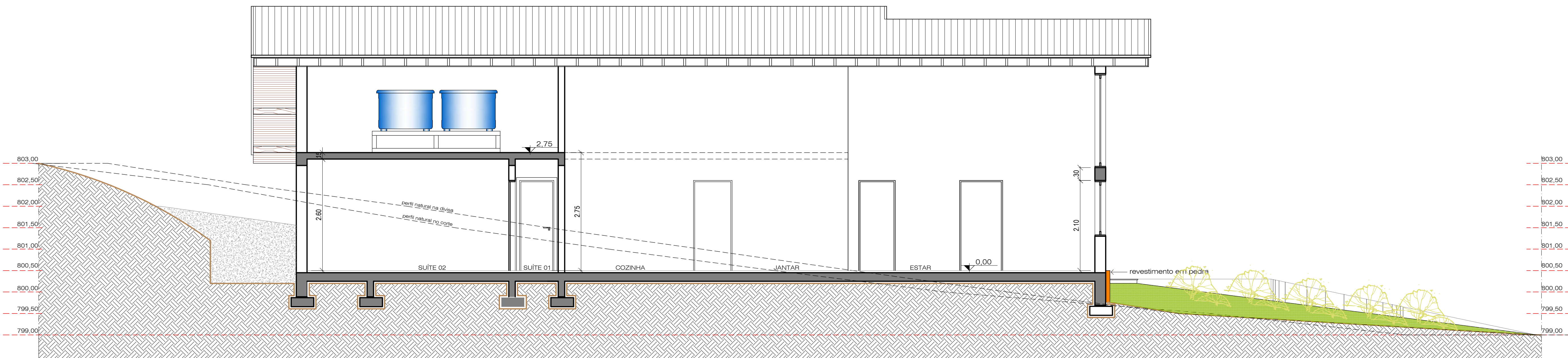
CORTE AA - esc.:1/50
