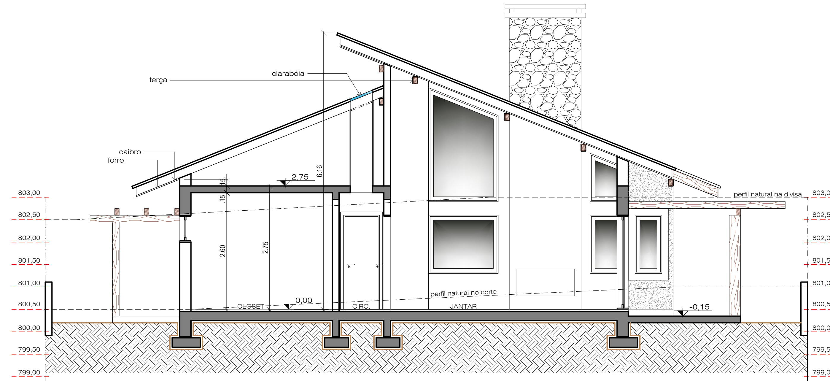
CORTE BB - esc.:1/50
