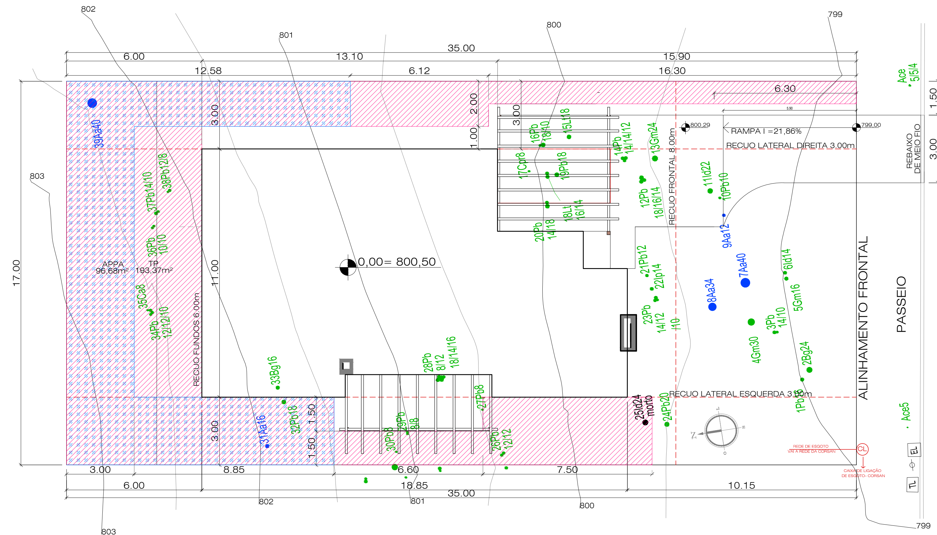
IMPLANTAÇÃO - esc.:1/100
